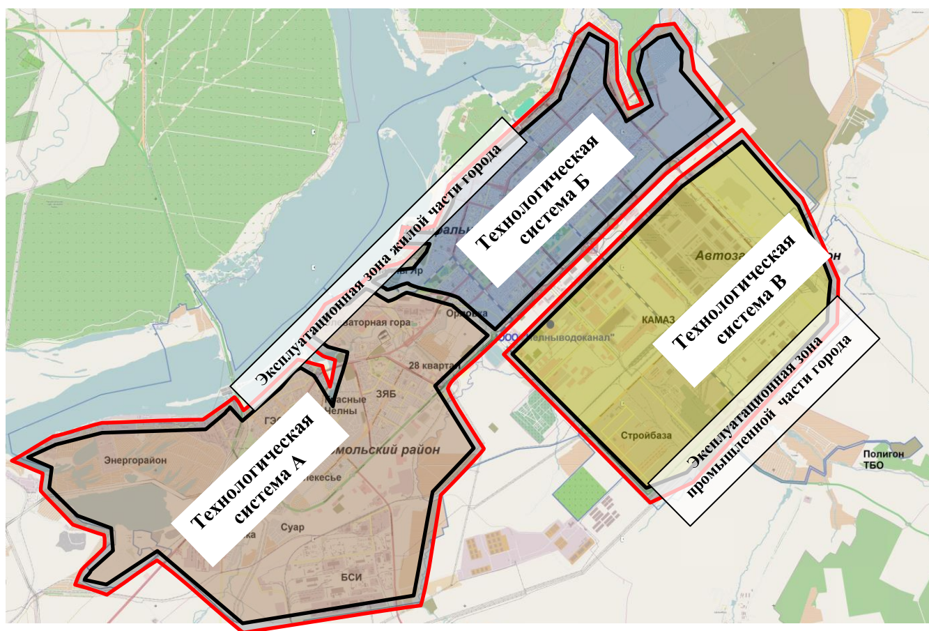
Рисунок 1 Эксплуатационные зоны и технологические системы водоснабжения и водоотведения
