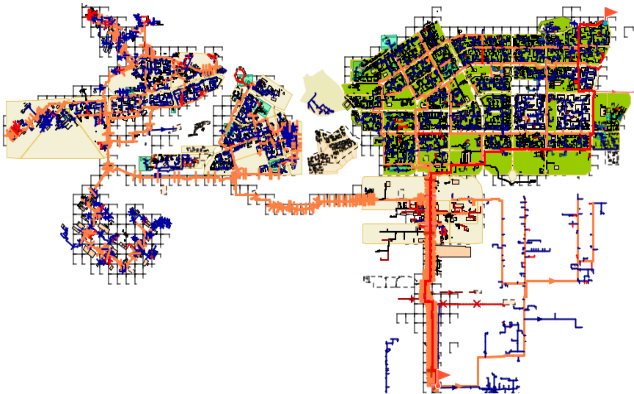
Рис. 6.6. Путь построения пьезометрического графика от «ТЭЦ» до конечного потребителя «ж.д. 50-20»
