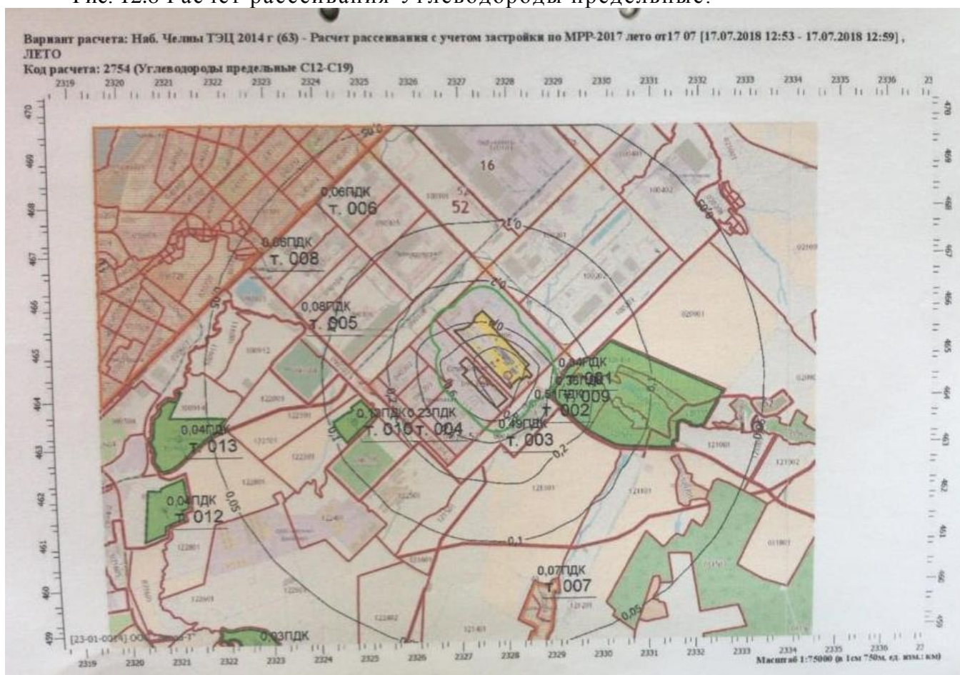
Рис. 12.8 Расчет рассеивания Углеводороды предельные.
